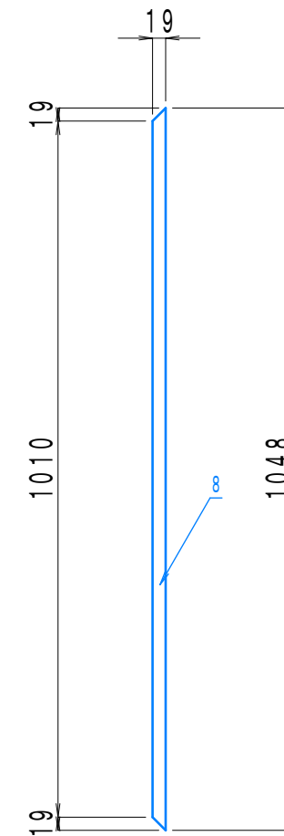
8 19x89x1048-4
