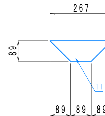
11 19x89x267-2
